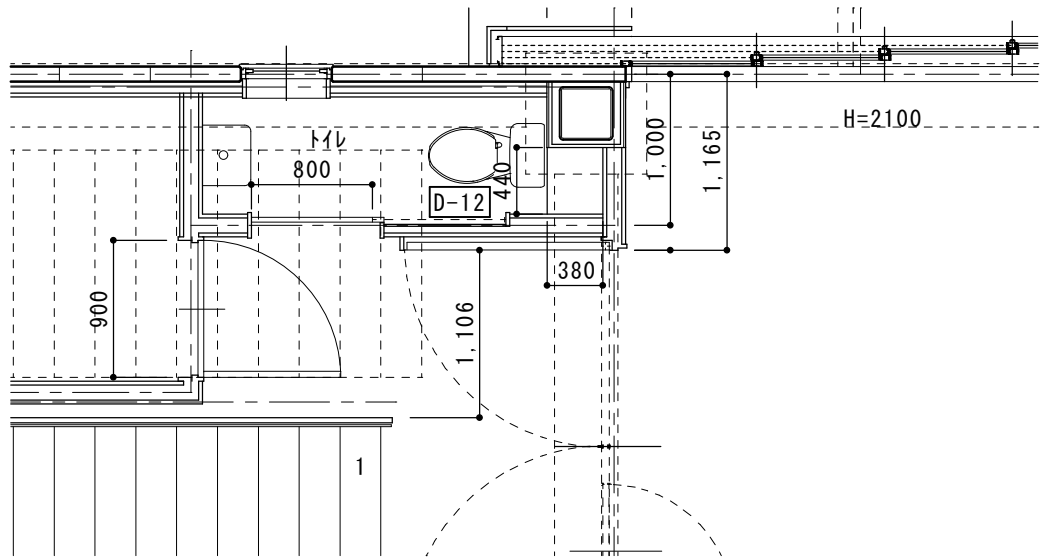
大人トイレ オープン棚 平面詳細図 1/50
